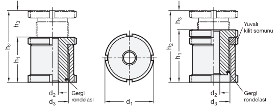
Tip AK (kilitleme somunu)
