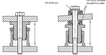
2 yuvartık dengeleme pulu İle Tip A (kilitleme somunsuz)
